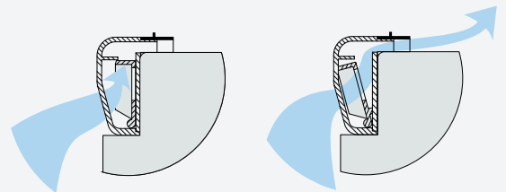
Volumenstrombegrenzung
