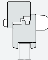
im Rahmen und im Flügel
