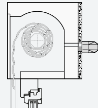
im Rollladenkasten mit Anputz- leiste und Schalldämmmodul
