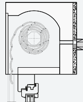
im Rollladenkasten mit Anputzleiste
